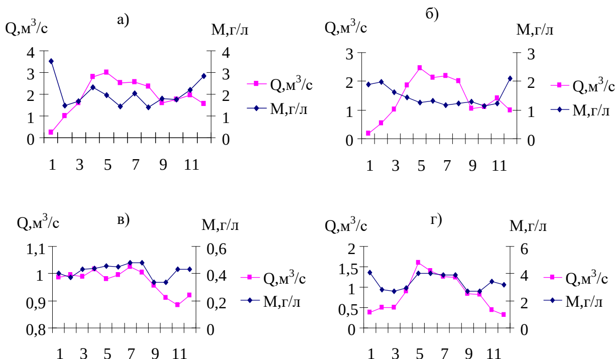
Рис. 3. Внутригодовые изменения расходов воды ( Q, \text{м}^3/\text{с} ) и минерализации ( M, \text{г/л} ) в крупных коллекторах Сурхандарьинской области в среднем за 2003-2006 гг.: а) МС; б) Ангор; в) К-2 Денов; г) К-2 Музрабод.
