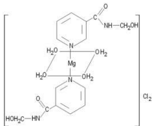
2-расм. Магдин \text{Mg}(\text{ОНК})_2\text{Cl}_2 \cdot 4\text{H}_2\text{O}
