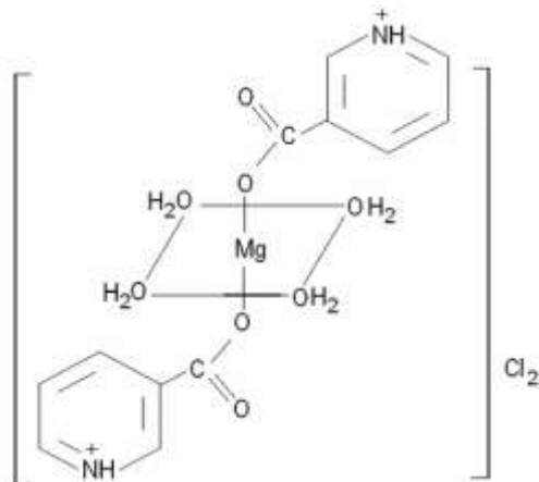
1-расм. Магнийком \text{Mg}(\text{HK})_2\text{Cl}_2 \cdot 4\text{H}_2\text{O}
