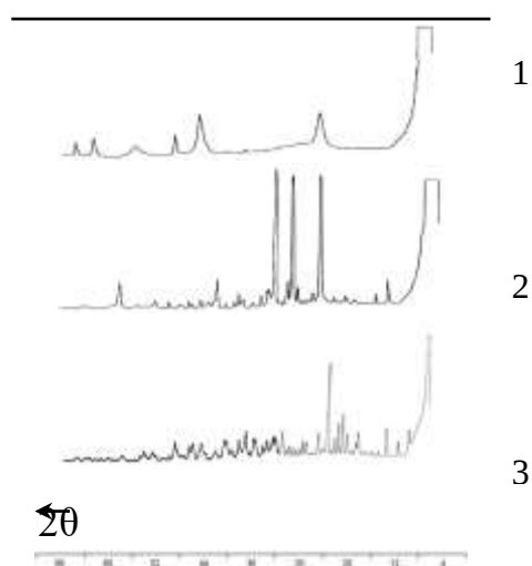
6- расм. 1 - \text{MgO} ; 2- ПН; 3- \text{Mg}(\text{ПН})_2\text{Cl}_2 рентгенограммалари
