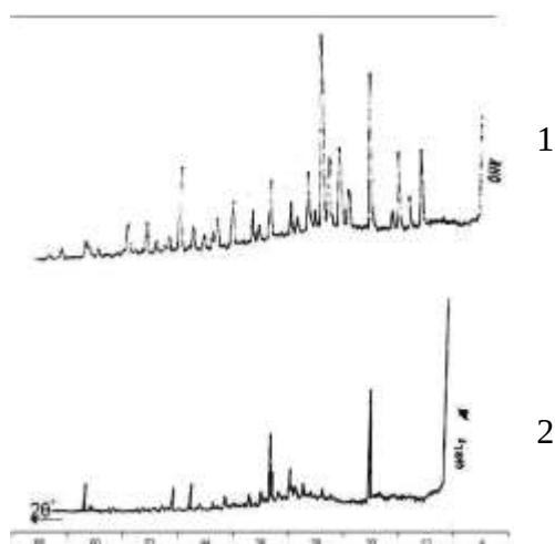
5-расм. 1-ОНК; 2 - \text{Mg}(\text{ОНК})_2\text{Cl}_2 \cdot 4\text{H}_2\text{O} рентгенограммалари
