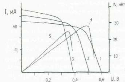
Рис.2. Нагрузочные ВАХ (1,2,3) и выходная мощность (4,5) фотоэлемента на основе аморфного кремния при T, \text{K}: 300 (1, 4); 350 (2); 400 (3, 5) .
