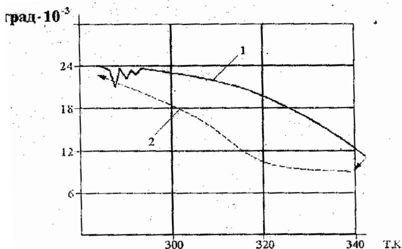
Рис. 6. Изменение величины эллиптичности адсорбированных ассоциатов феофитина при их нагревании (1) и охлаждении (2).
