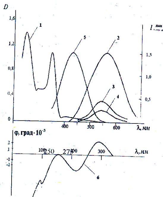
Рис.2. Спектр поглощения (1), люминесценции (2,4), возбуждения люминесценции (5) и дисперсии оптического вращения (6) рутина в диметилсульфоксиде. Длины волн возбуждения люминесценции 450 (2), 362(3) и 300 нм (4). Длина волны регистрации люминесценции 540 нм C=0,56 г/л. l=0,1 см.
