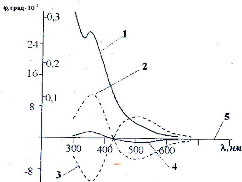
Рис. 5. Спектры поглощения (1) не гиротропного поворота плоскости поляризации адсорбированных ассоциатов рутина при повороте кюветы на 45^{\circ} (2), -45^{\circ} (3), 5^{\circ} (4) вокруг светового пучка, сумма спектров 2 и 3 (5)
