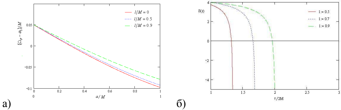
Рис.3. Зависимость знака а) \Omega_F - \omega_3/M от параметра a/M и
