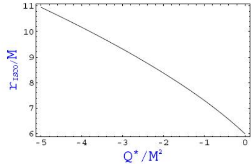
Рис.2. Зависимость минимального радиуса круговой орбиты (а) и радиуса СКО (б) вокруг ЧД от бран заряда.
