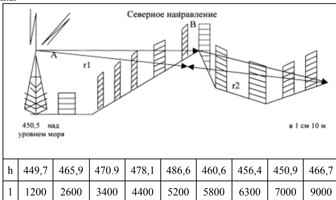
Рис. 4. Профиль передачи радиоволн в северном направлении
