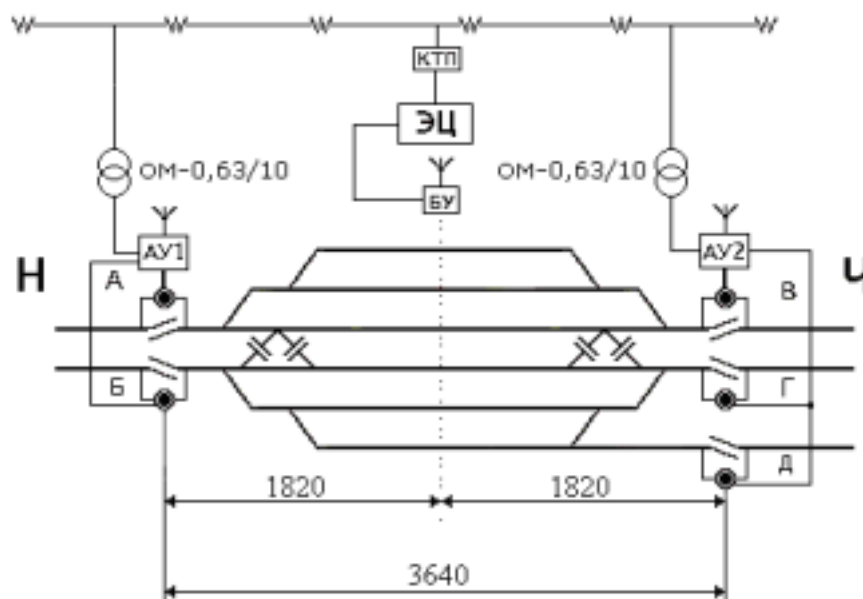
Рис. 2. Схема электроснабжения станции
