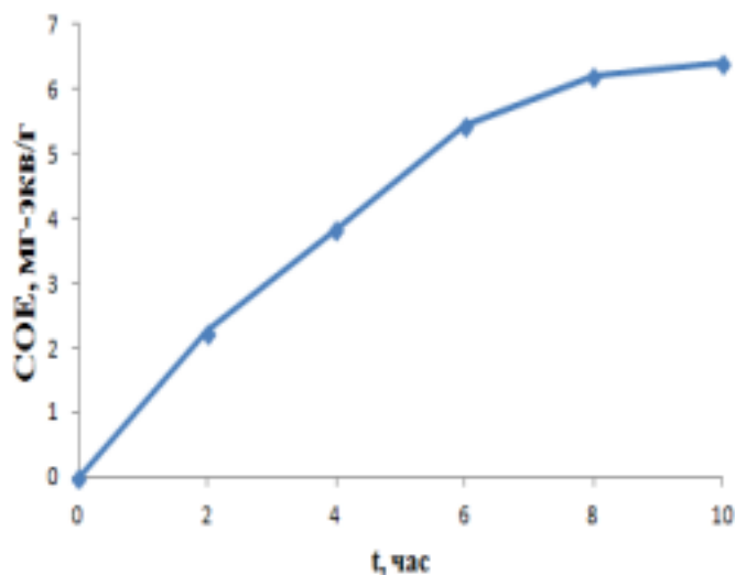
Рис. 2. Зависимость СОВ анионита ППЭ-1 от продолжительности времени реакции ( C_{\text{ППЭ}}=80\% ; T_{\text{сорбции}}=100^{\circ}\text{C} ; T_{\text{дозревания}}=150^{\circ}\text{C} ).
