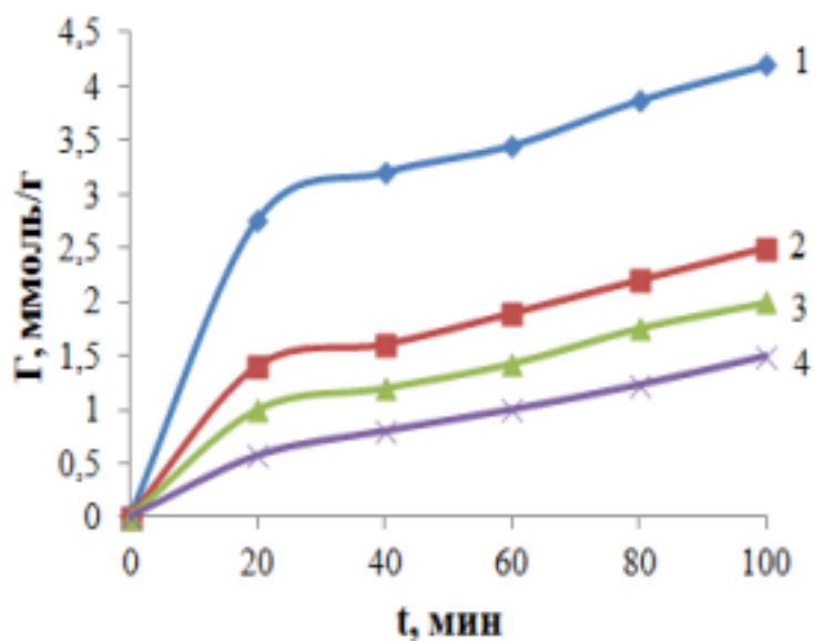
Рис. 3. Кинетика поглощения йода анионитом ППЭ-1. 1, 2, 3, 4-концентрация йода соответственно 0,05; 0,025; 0,01; 0,0075 моль/л, температура-313К
