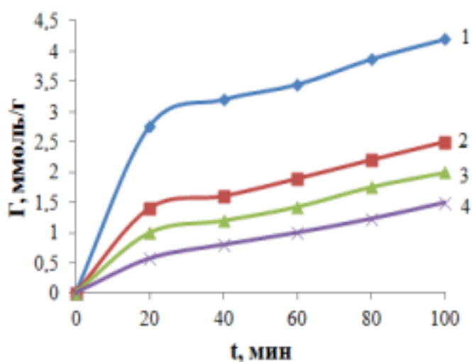
3-расм. ППЭ-1 анионитига йодни ютилиш кинетикаси. 1, 2, 3, 4- йодни бошлангич концентрацияси мос равишда 0,05; 0,025; 0,01; 0,0075 моль/л, ҳарорат-313К
