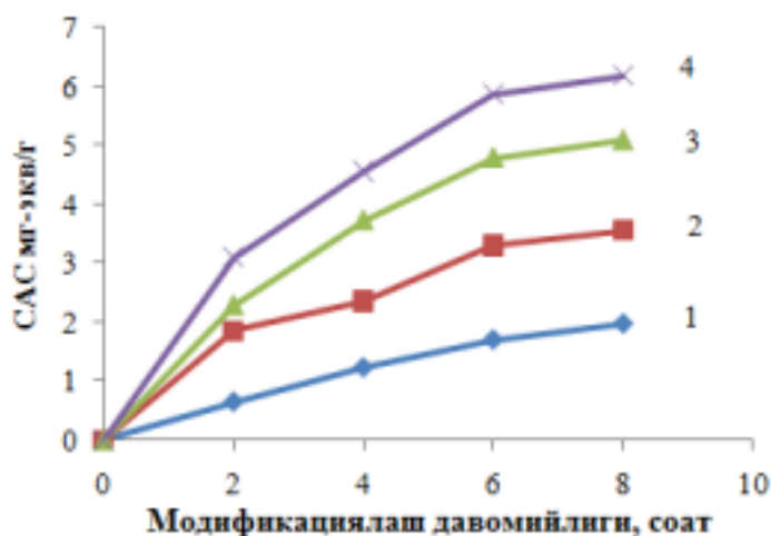
2-расм. Анионитнинг статик алмашиниш сизимини модификациялаш давомийлигига боғлиқлиги. (1, 2, 3, 4- реакция ҳарорати мос равишда 393, 403, 413, 423K).
