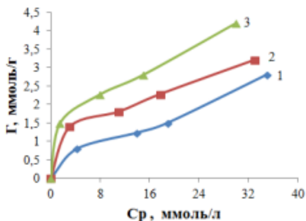
4-расм. ППЭ-1 анионитига йодни турли ҳароратлардаги ютилиш изотермаси, 1, 2, 3 ҳарорат мос 293, 303, 313K.
