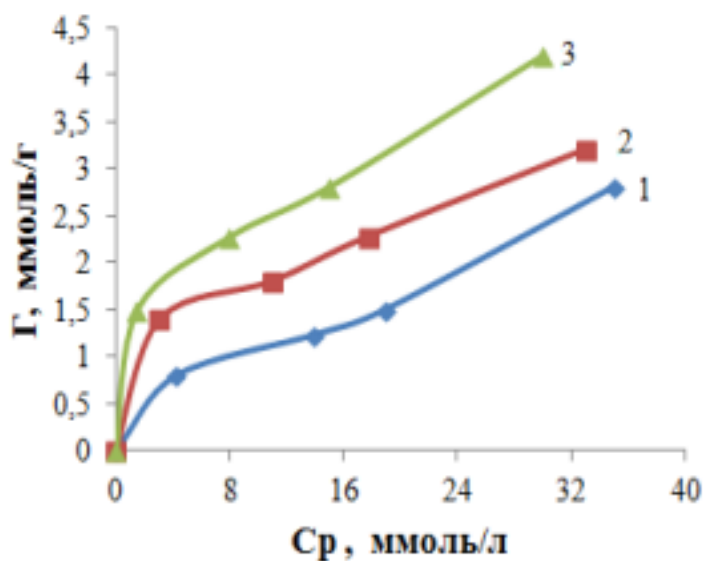
Рис. 4 Изотермы сорбции йода анионитом ППЭ-1 при различных температурах. 1, 2, 3 температура соответственно 293, 303, 313К
