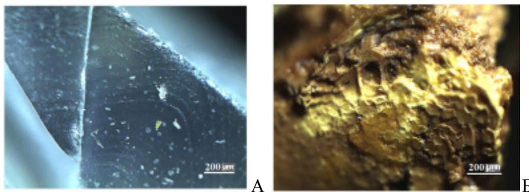
Рис. 1. Вид в оптическом микроскопе гранул поливинилхлорида(А) и анионита (Б)
