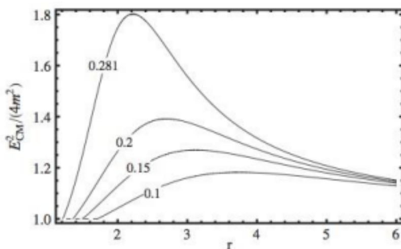
6-расм. \omega = 0,1, 0,15, 0,2, ва 0,281 қийматлар учун Кепплер орбитада ҳаракатланаётган ва радиал йўналишда келаётган икkitа зарраларнинг масса маркази энергиясининг радиал ўзгариши
