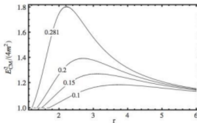
Рис. 6. Радиальная зависимость энергии центра масс сталкивающихся радиально падающих и вращающихся по круговой Кеплеровской орбите частиц для различных значений параметра \omega = 0,1, 0,15, 0,2 , и 0,281
