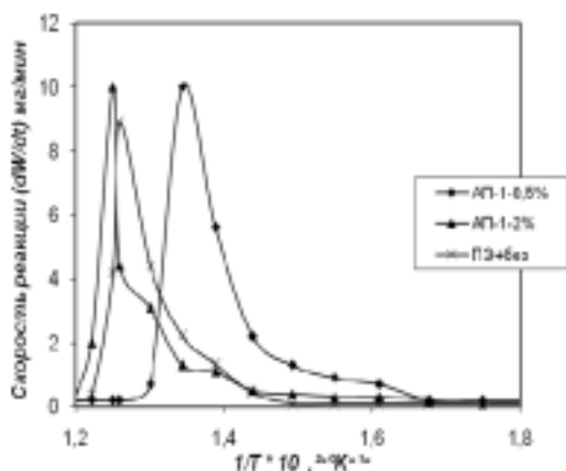
Рис.4. Сравнение зависимостей производных кривых при деструкции полиэтилена с модифицированными полиэти
