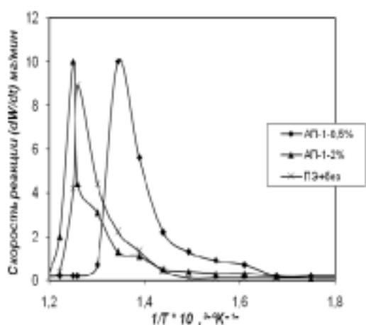
4-расм. Модификацияланган полиэтиленларнинг вакуум шароитида полиэтиленнинг деструкциясида ҳосилалли эгри чизиклари боғлиқлигининг таққосланиши
