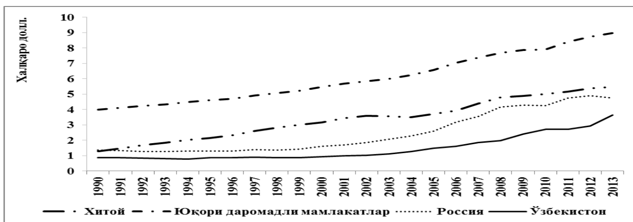
2-расм. ЯИМ энергия сифимдорлиги (ҳар бир килограмм нефть эквивалентига тўғри келувчи ХҚП бўйича ЯИМ) [13]
