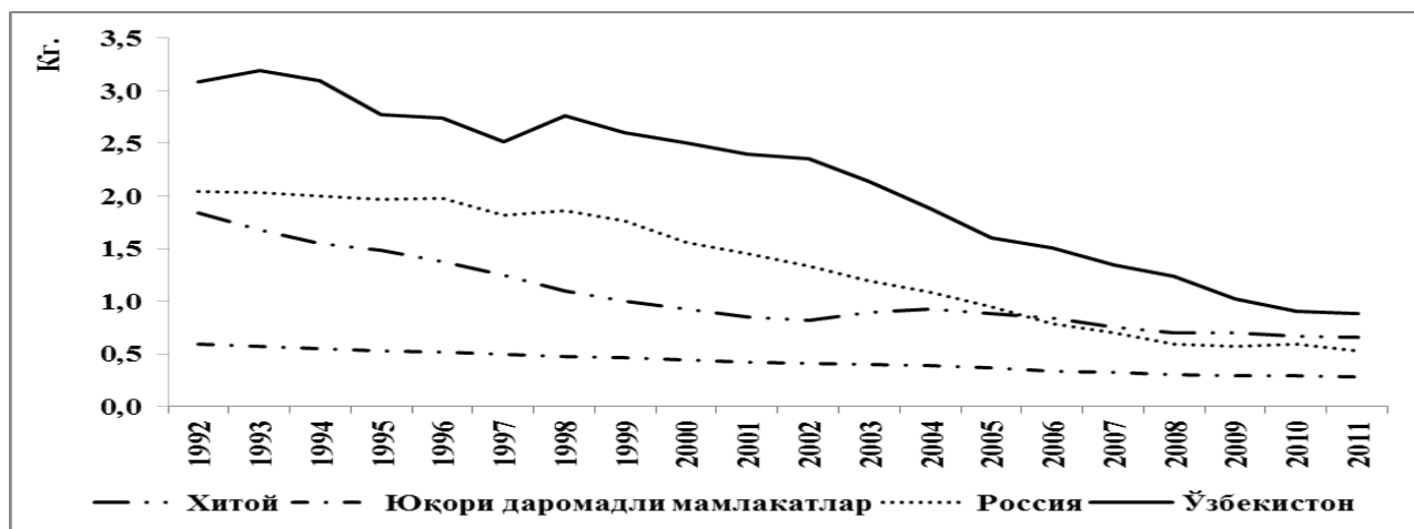
3-расм. CO2 чиқиндиси (ХҚП бўйича ЯИМ ҳар бир АҚШ доллариға тўғри келувчи CO2 чиқиндиси) [14]
